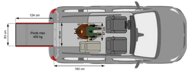
VERSION FIXE 3 PLACES + 1 PERSONNE EN FAUTEUIL ROULANT
