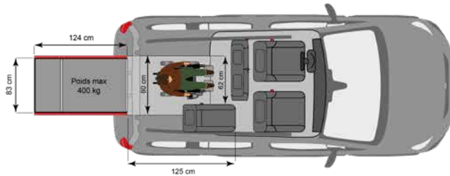
VERSION D'ORIGINE 3 PLACES + 1 PERSONNE EN FAUTEUIL ROULANT
