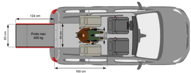
VERSION FIXE 4 PLACES + 1 PERSONNE EN FAUTEUIL ROULANT
