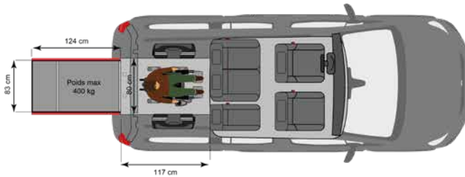
VERSION D'ORIGINE 5 PLACES + 1 PERSONNE EN FAUTEUIL ROULANT
