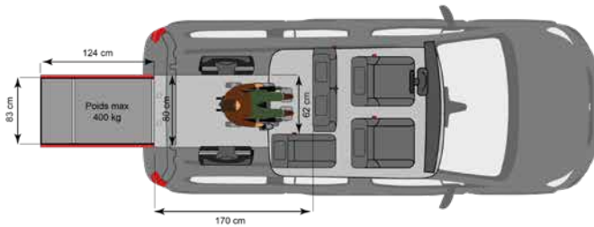
VERSION D'ORIGINE 3 PLACES + 1 PERSONNE EN FAUTEUIL ROULANT
