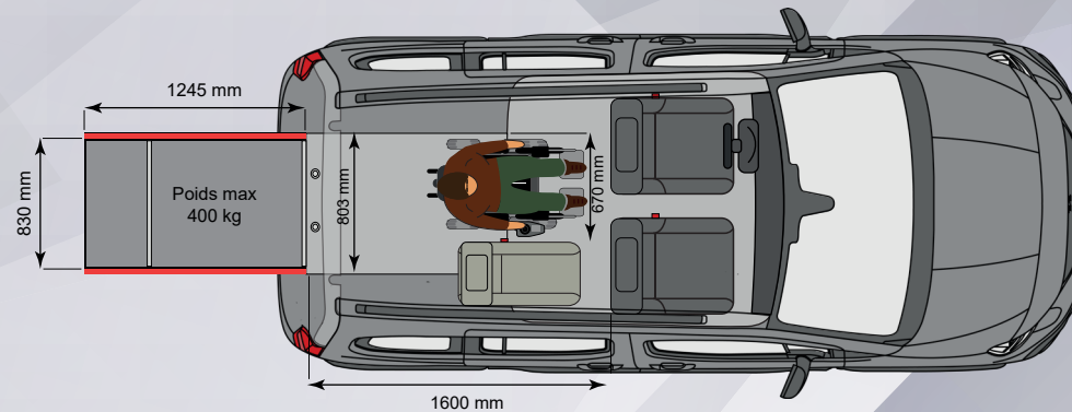
VERSION SIÈGE FIXE, 3 PLACES + 1 FAUTEUIL
