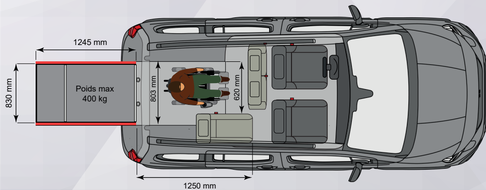
VERSION BANQUETTE D'ORIGINE, 3 PLACES + 1 FAUTEUIL
