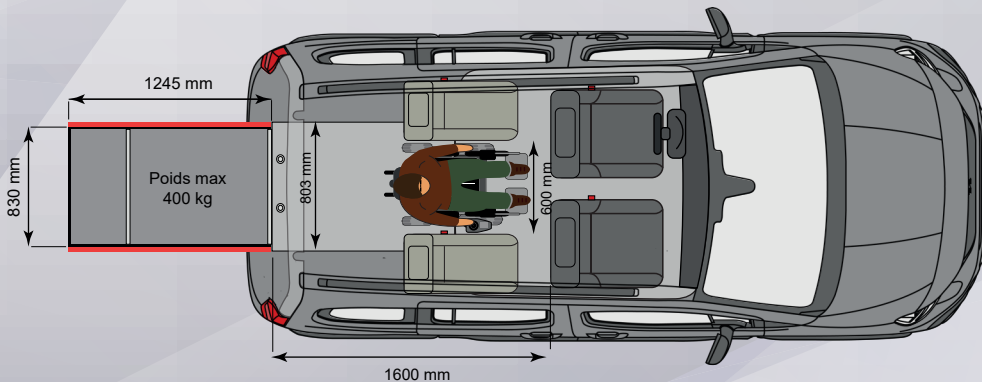
VERSION SIÈGES FIXES, 4 PLACES + 1 FAUTEUIL
