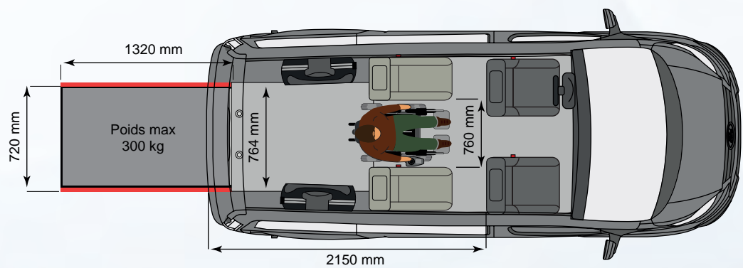
VERSIONS 4 PLACES + 2 SIÈGES STRAPONTINS + 1 FAUTEUIL
