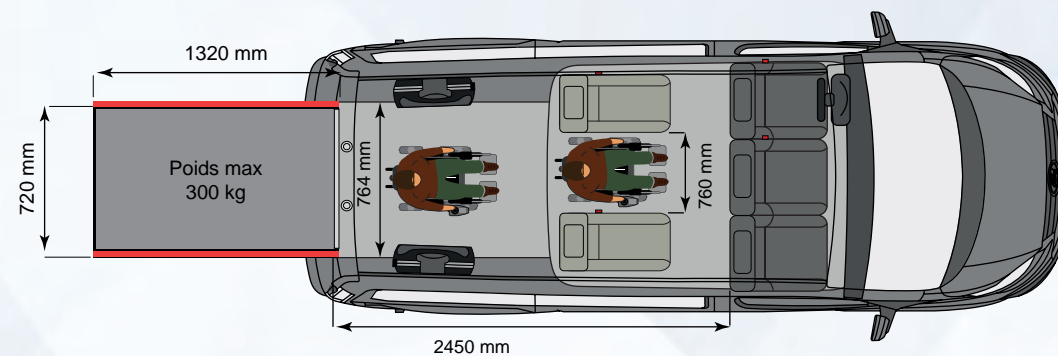
VERSION 5 PLACES + 2 FAUTEUILS
