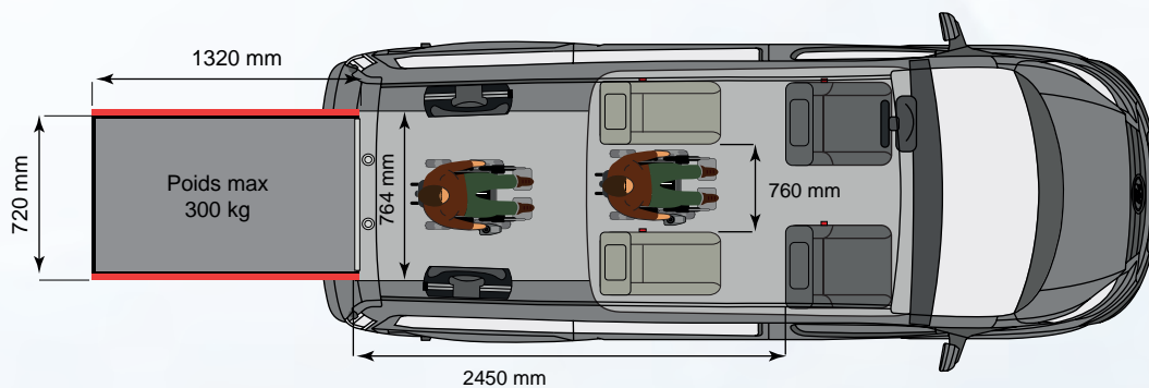
VERSION 4 PLACES + 2 FAUTEUILS
