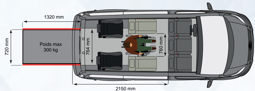
VERSION 5 PLACES + 2 SIÈGES STRAPONTINS + 1 FAUTEUIL
