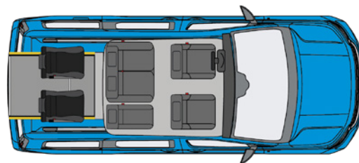
VERSION D'ORIGINE 7 PLACES (DONT 2 STRAPONTINS)
