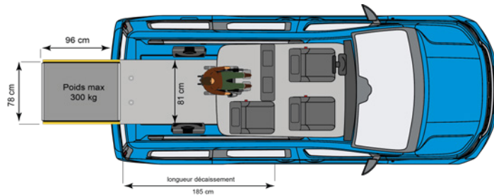
VERSION D'ORIGINE 2 PLACES + 1 FAUTEUIL ROULANT (BANQUETTE ARRIÈRE ET 2 STRAPONTINS REPLIÉS)
