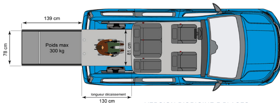
VERSION D'ORIGINE 5 PLACES + 1 PERSONNE EN FAUTEUIL ROULANT (DONT 2 STRAPONTINS REPLIÉS)
