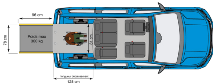
VERSION D'ORIGINE 5 PLACES + 1 PERSONNE EN FAUTEUIL ROULANT (DONT 2 STRAPONTINS REPLIÉS)
